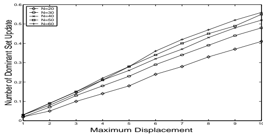
Fig. 6. Dominant set updates, tx\_range=30
